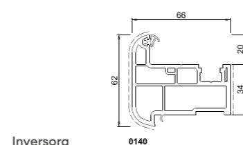
Inversora
